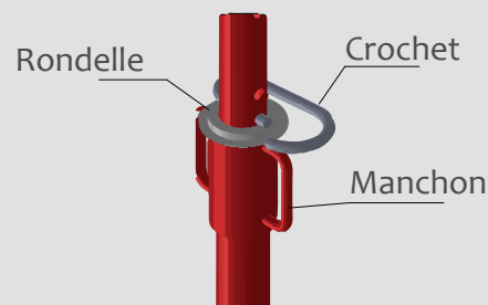
Manchon Soudé
