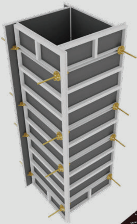
Panneaux Phénoliques
