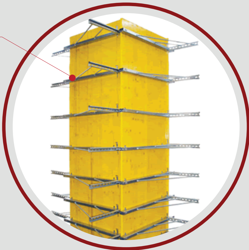
Cravate pour pilier
