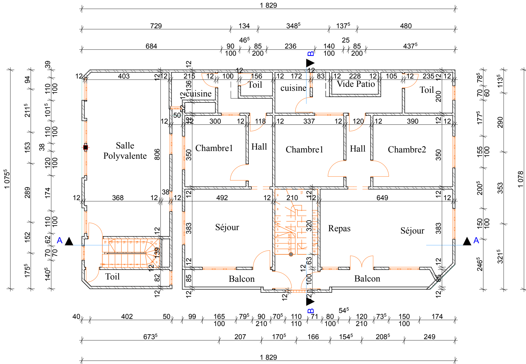
VUE EN PLAN DE RECOLLEMENT DU R+1 ECH:1/100
